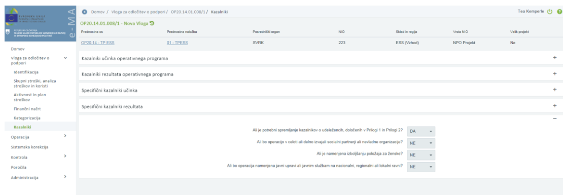
Slika 54: Kazalniki
