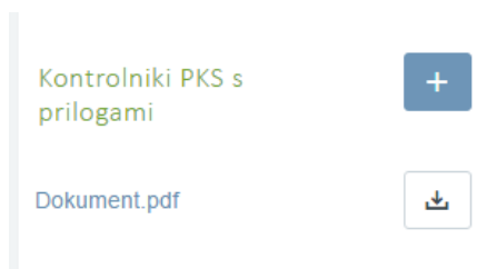
Slika 273: Dodajanje priloge
