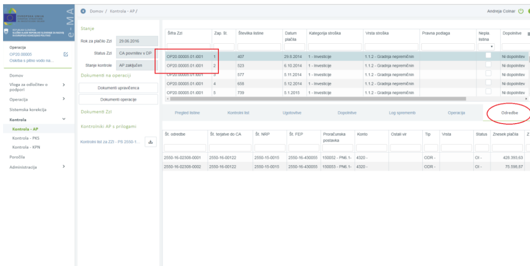
Slika 261: Zavihek Odredbe
