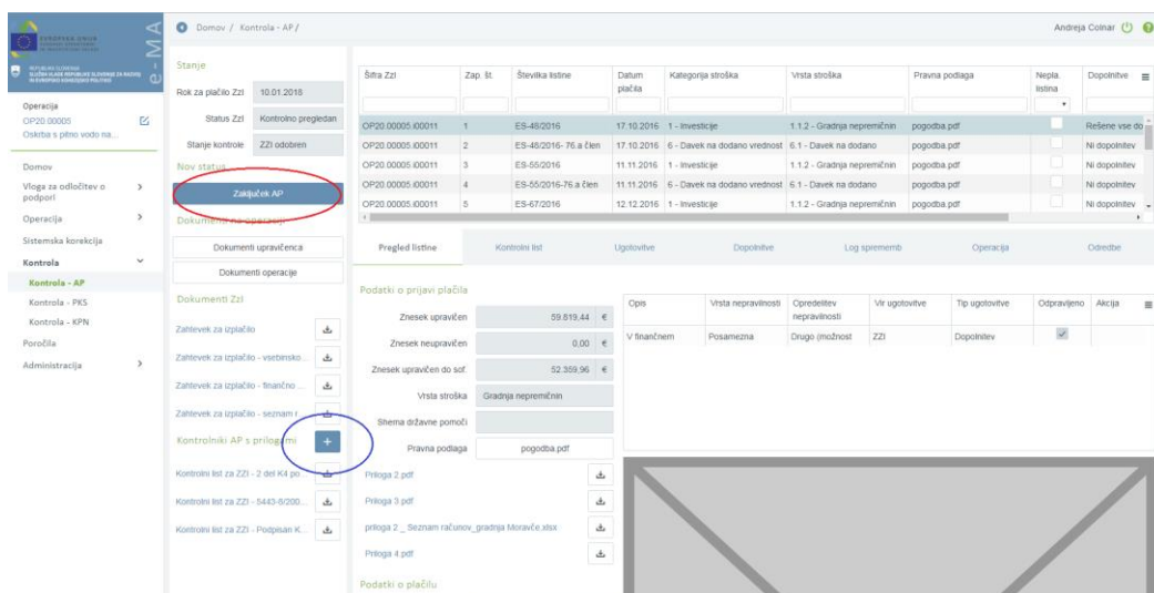
Slika 255: Zaključek AP
